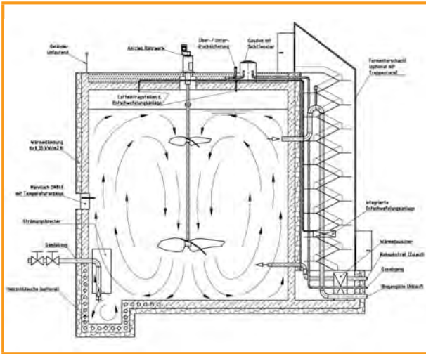
Şekil 3.33: Eksenel karıştırıcılar [ENTECH Environmental Technology Umwelttechnik GmbH]
