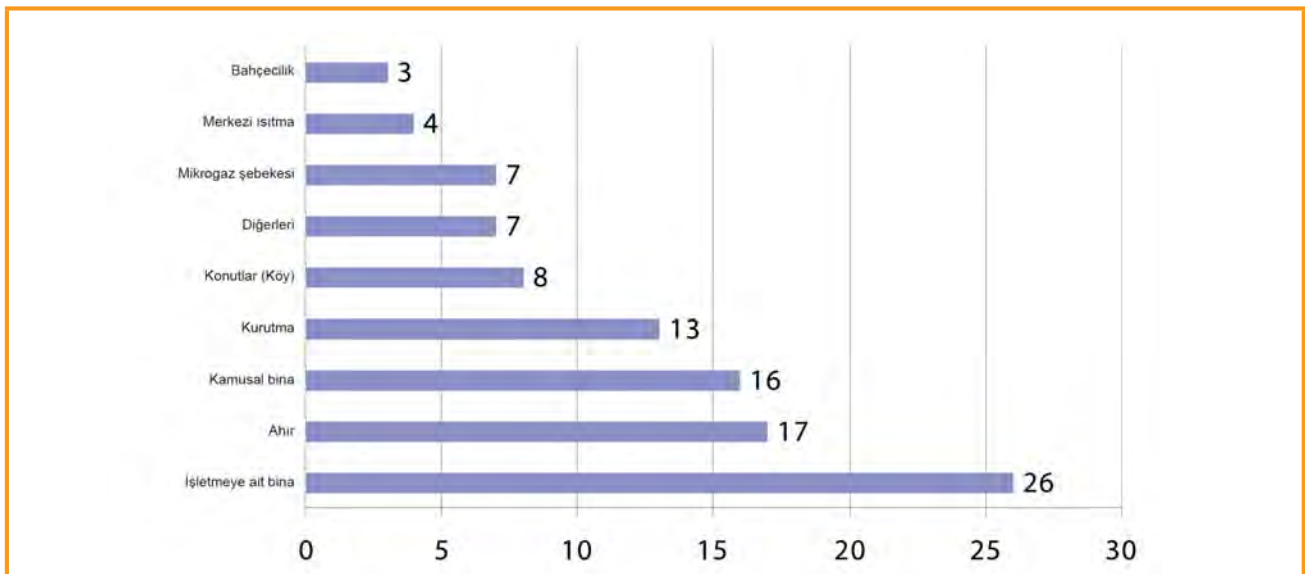
Şekil 8.1: KWK prosesli biyogaz tesislerinde atık ısı faydalanım yolları [8-7]
