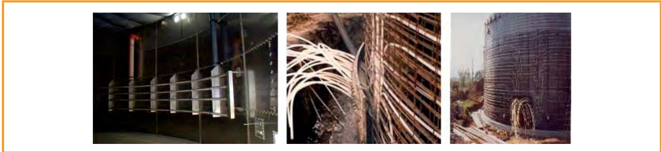
Şekil 3.37: Fermentöre döşenmiş paslanmaz çelik ısıtıcı borular (iç tarafta) (solda); fermentör duvarına ısıtıcı hortumlarının montajı (sağda) [Biogas Nord GmbH; PlanET Biogastechnik GmbH (sağ)]
