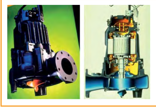
Şekil 3.9: Parçalama ve taşıma düzeneği kombinasyonu olarak rotorda kesici kenarları bulunan dalgiç pompa [ITT FLYGT Pumpen GmbH]
