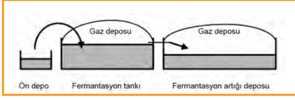
Şekil 3.2: Depolamalı-akışlı yöntem
