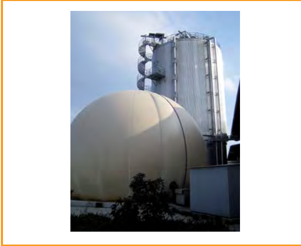
Şekil 3.40: Bağımsız çift membranlı depo örneği [Schüsseler, FNR]
