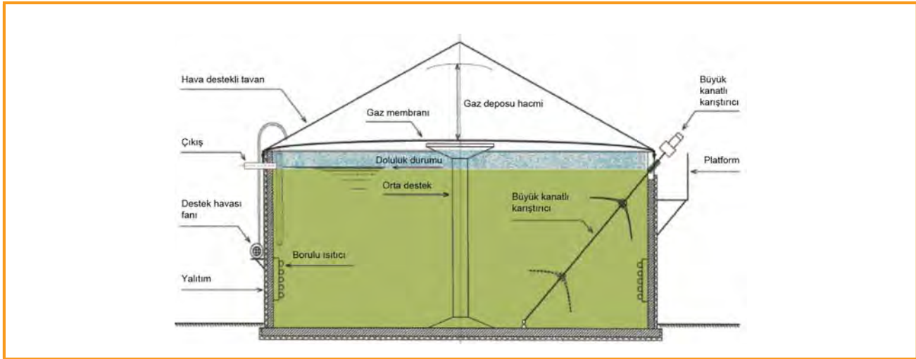
Şekil 3.22: Tam karışımli fermentör, uzun akslı karıştırıcı ve diğer yapılarla birlikte [Anlagen- und Apparatebau Lütke GmbH]
