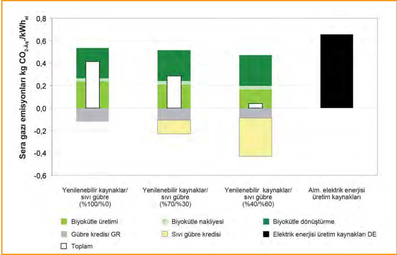
Şekil 12.2: Model biyogaz tesislerinden sera gazı emisyonları (kg CO 2-Aq ./kWh el ) Alman elektrik enerjisi üretim kaynaklarına kıyasla (GR = Fermantasyon artığı) [12-5]
