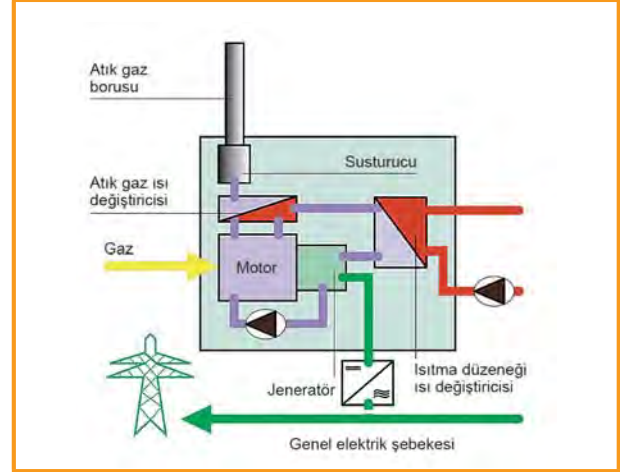
Şekil 6.4: Bir kojenerasyon santralinin yapısı [ASUE]
