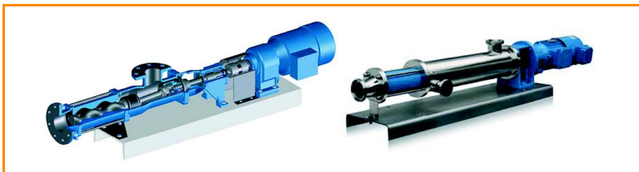
Figura 3.12: Bomba de tornillo de rotor único excéntrico [LEWA HOV GmbH + Co KG]
