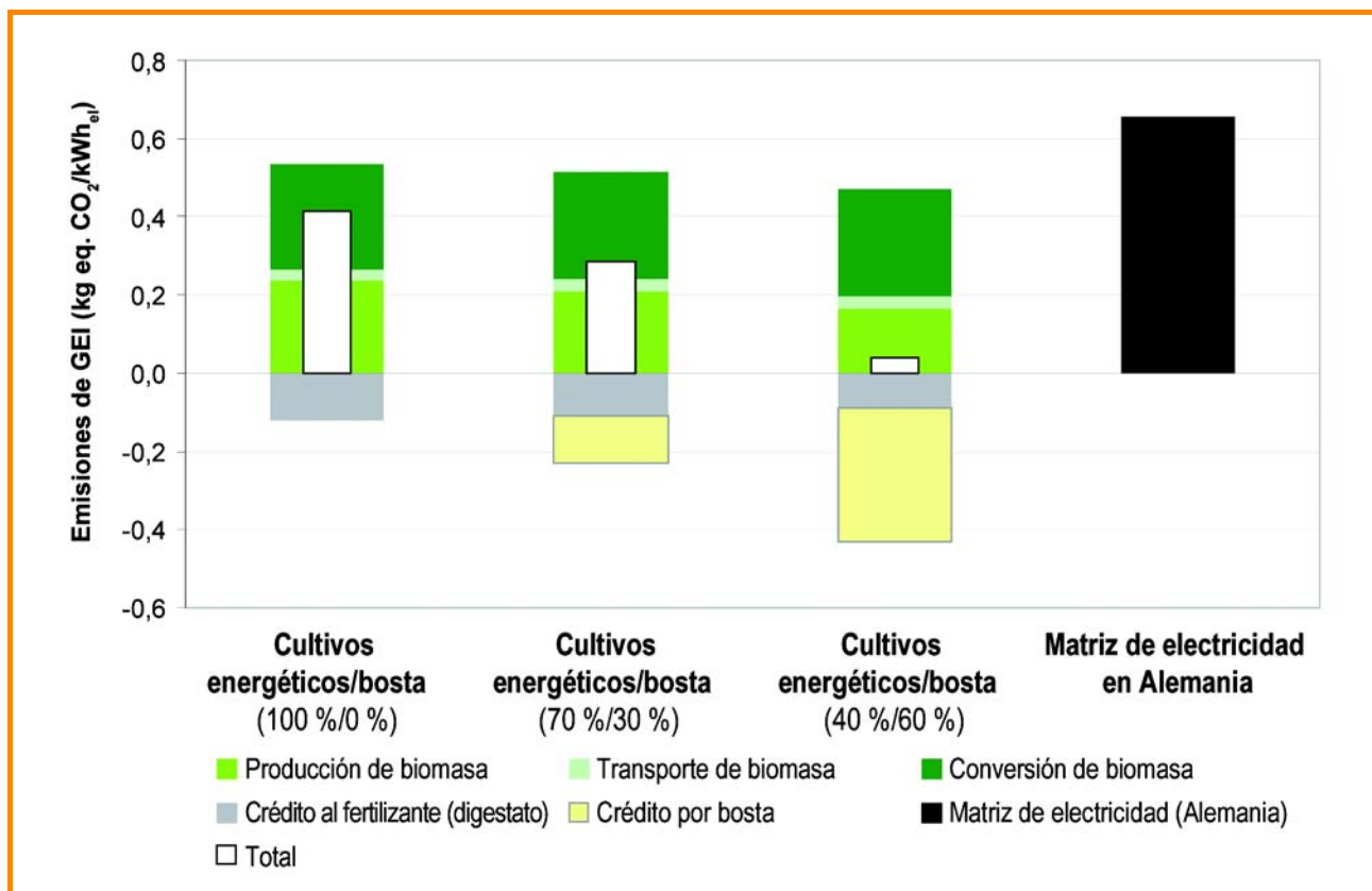
Figura 12.2: Emisiones de gas de efecto invernadero ( \text{kg CO}_2 equivalente /\text{kWh}_{el} ) provenientes de las plantas de biogás modelo comparadas con mezclas de electricidad en Alemania [12-5]
