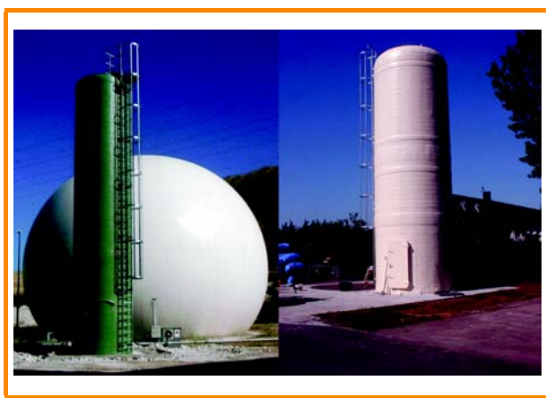
Figura 6.2: Torres externas de desulfuración biológica, a la derecha de un contenedor de gas [S&H GmbH & Co. Umweltengineering KG].
