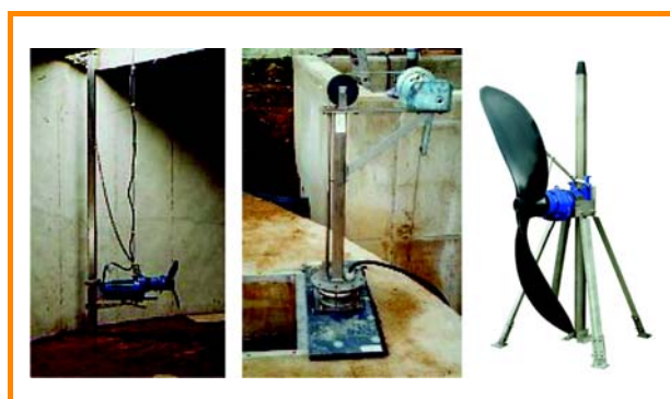
Figura 3.31: Propulsor SMA (izquierda), sistema de tubo guía (centro), rotor de cuchillas grandes SMA (derecha) [Agrartechnik Lothar Becker (izquierda, centro), KSB AG]
