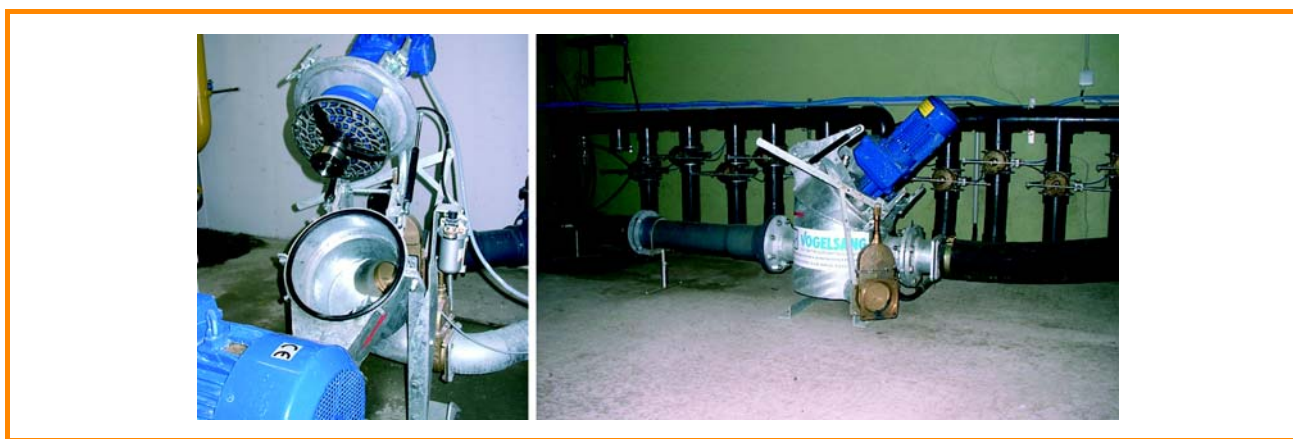
Figura 3.8: Triturado de sustrato en tuberías (con dispositivo de triturado de placa perforada) [Hugo Vogelsang Maschinenbau GmbH]
