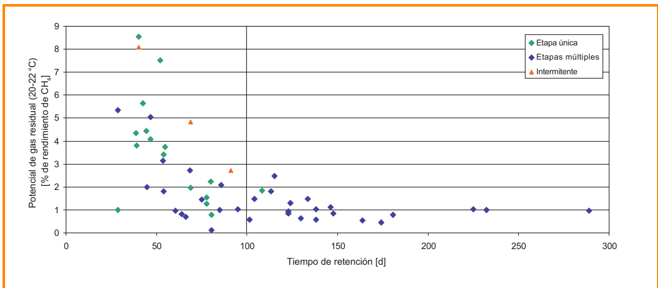
Figura 10.1: Correlación entre el potencial relativo de gas residual a 20 - 22 °C y el tiempo de retención hidráulica [10-8]
