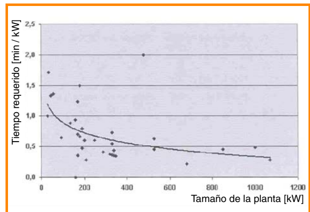
Figura 9.4: Tiempo de trabajo requerido para la supervisión de una planta [9-4]
