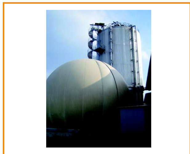
Figura 3.40: Ejemplo de un tanque de almacenamiento de láminas plásticas independientes con dos espesores de láminas plásticas [Schüsseler, FNR]
