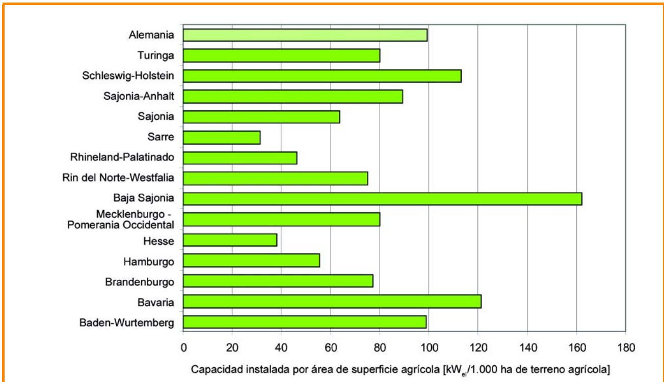
Figura 12.4: Capacidad eléctrica instalada en relación con el área de terreno agrícola [kW el /1.000 de terreno agrícola] en los estados federados alemanes (según los datos de [12-3], [12-6])
