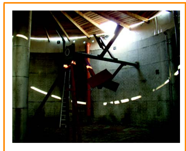
Figura 3.34: Agitador de paletas [PlanET GmbH]
